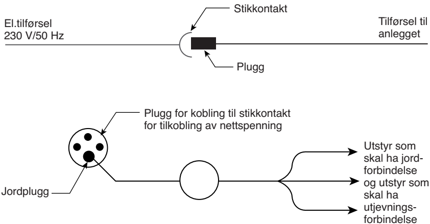
Figur 21.1 Eksempel på kontinuitetsmåling
