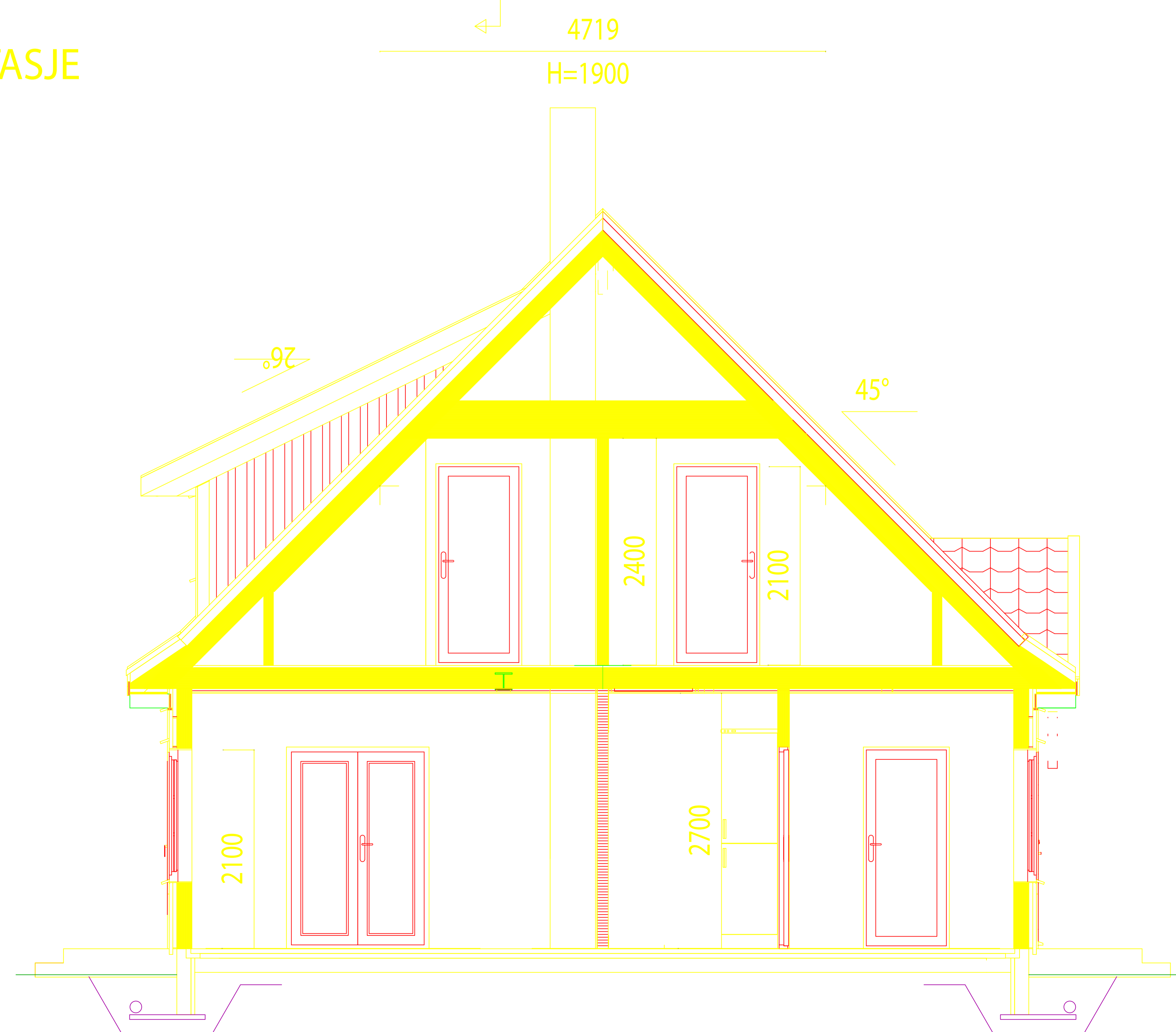
SNITT A-A
