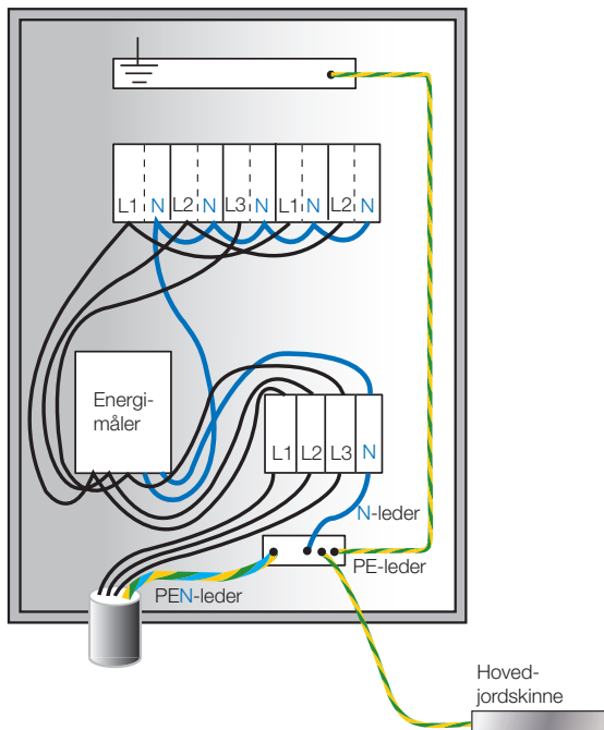
Figur 10.4 Felles jord og nøytralleader må splittes i fordelingskapet
