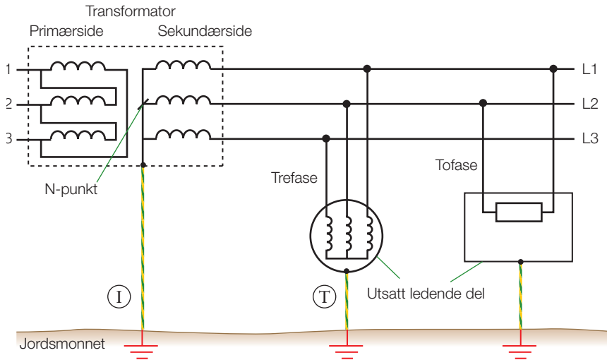
Figur 10.1 Prinsippskisse for TT-system
